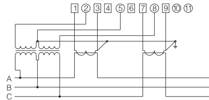
DSSD型三相三线电子式多功能电能表接线图(电流、电压互感器式)
