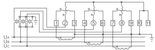
DTSD型三相四线电子式多功能电能表接线图(电流、电压互感器式)
