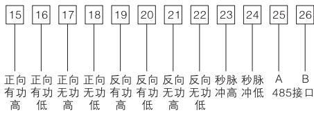
辅助端子接线图
